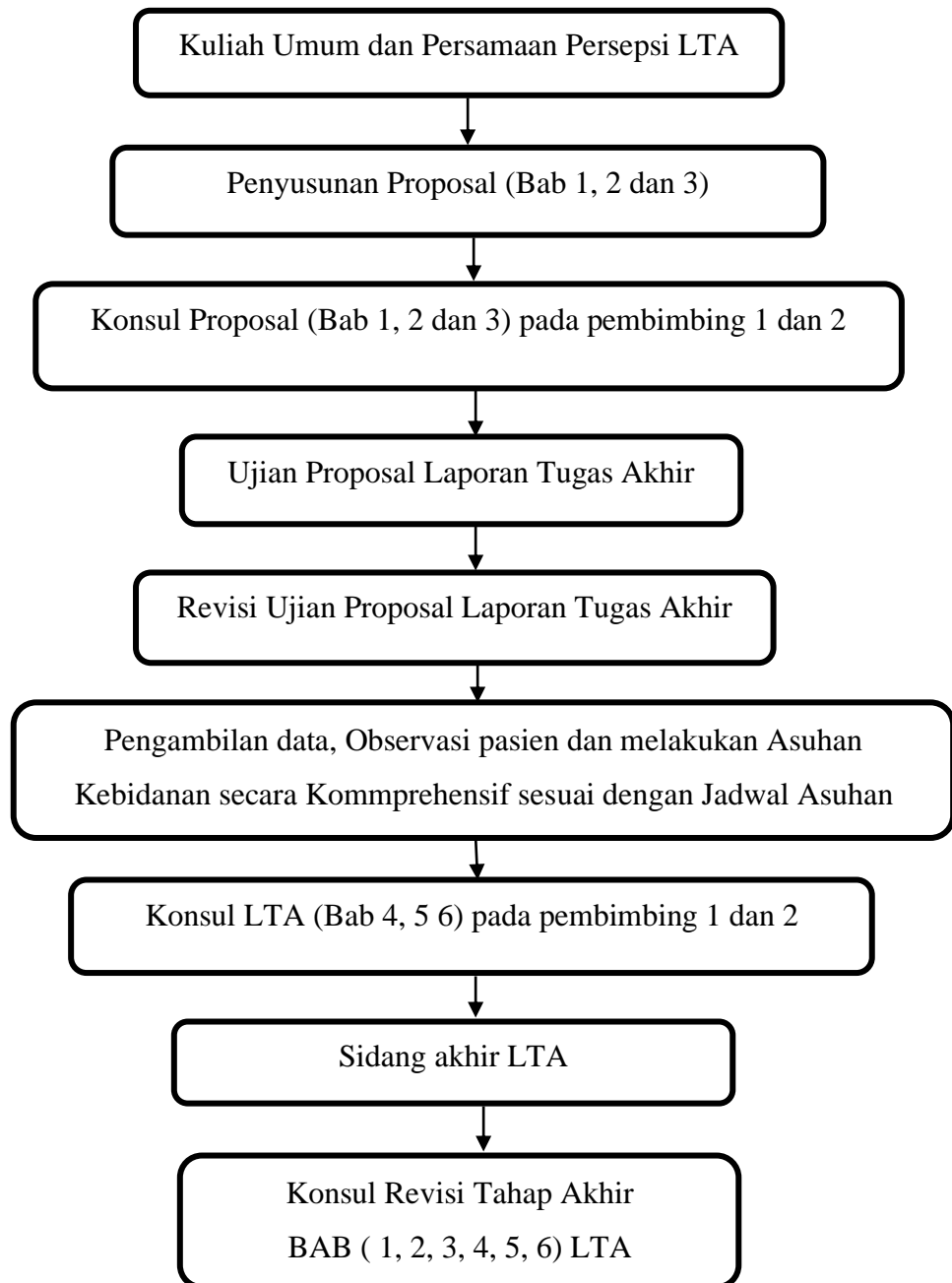
Gambar 3.2 Kerangka Kerja
